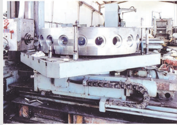
ساخت کامل قطعه FANCOOLER مجتمع فولاد مبارکه
