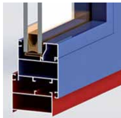
سیستم پنجره آلدوکس سبک طرح ایران سری AH45L
