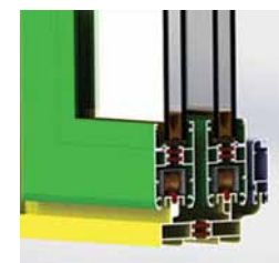
سیستم پنجره ترمال بریک سری TS77
