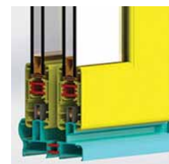
سیستم پنجره ترمال بریک سری TS94
